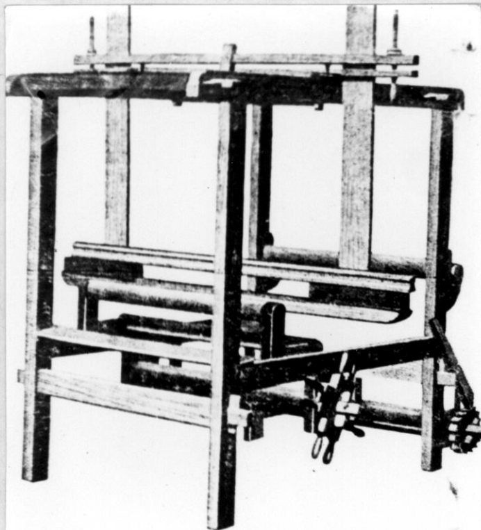
Kézi szövőszék facsapos hengerekkel és fa- csapágyakkal
